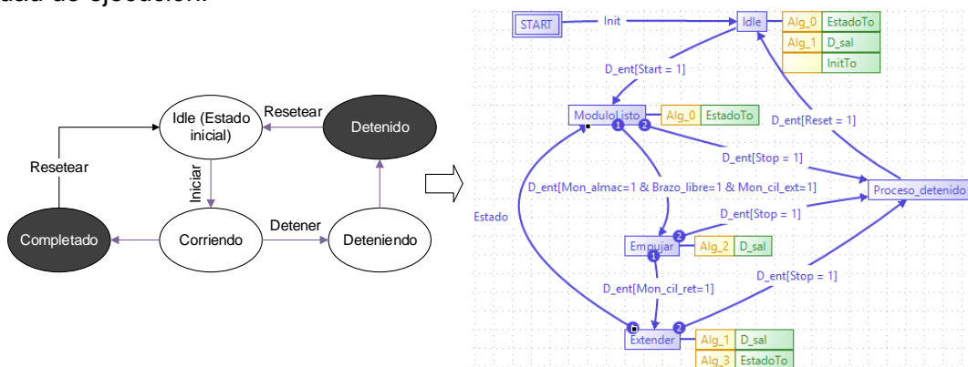
Figura 13. Estados ISA-88 de la estación MPS combinados al ECC
