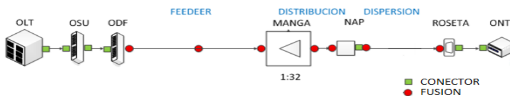
Figura 2. Diagrama, presupuesto óptico (Norma técnica de diseño de ODN, CNT, 2012).
