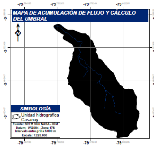
Figura 8. Acumulación de flujo y cálculo del umbral.
